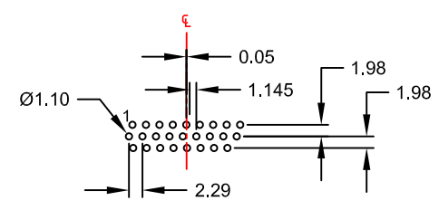
26-contact
